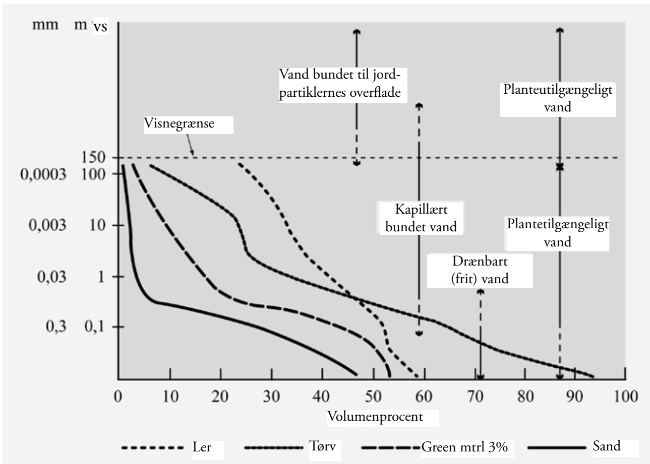
Figur 3. Retentionskurver for tørv, ler og greenmateriale efter USGA-specifikation (30 cm vækstlag over drængrus) med 3 vægtprocent organisk materiale samt sand. På den lodrette akse vises de vandbindende kræfter i enheden meter vandsøjle og hvilke porestørrelser disse kræfter svarer til i mm. Den vandrette akse viser volumenindholdet af vand, luft og faste partikler. Sammenlign med tekst og figur på side 10.
